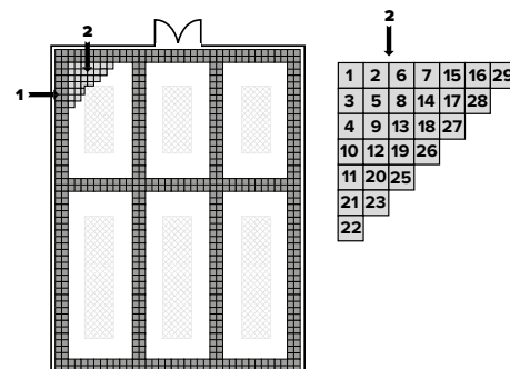
Abb. 6 : Verlegung um feste Objekte herum – das Verfahren zum Verlegen von Fliesen
